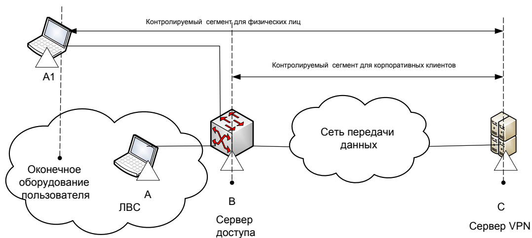
а) схема установки измерительных зондов в проводных сетях передачи данных
